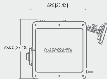
侧视图
