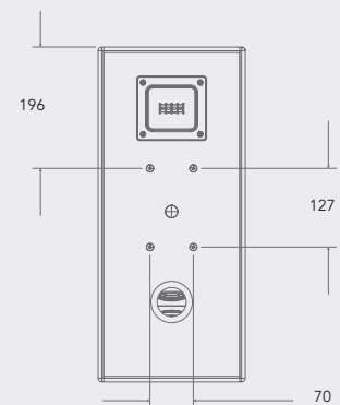
Вид сзади
