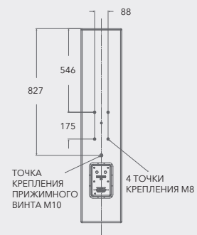
Вид сзади
