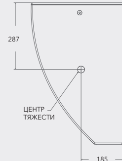
Вид сверху
