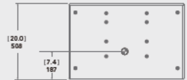
后视图
