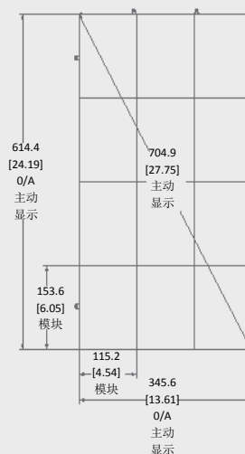
背视图
