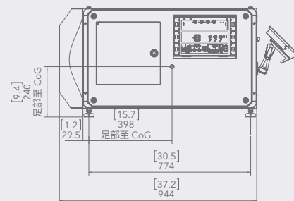
俯视图
