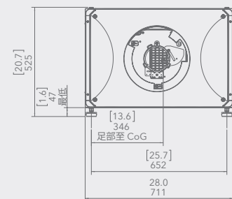
侧视图
